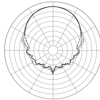
Horizontal 8000 Hz 1/3 Octave Polars
