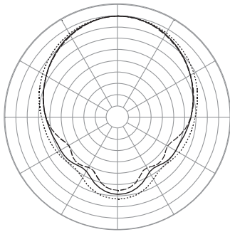
Horizontal 2000 Hz 1/3 Octave Polars
